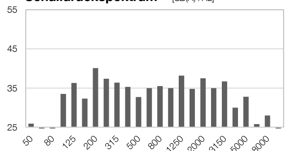
Schalldruckspektrum 5) [dB(A) /Hz]
