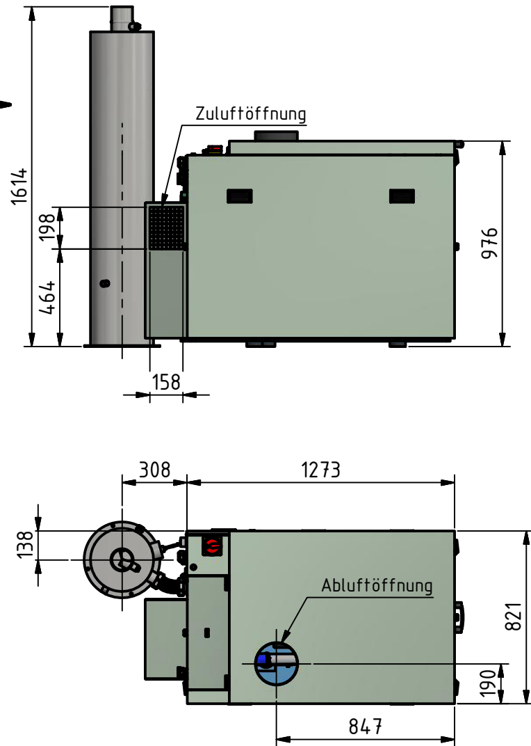
Ansicht A
