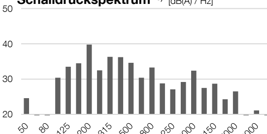
Schalldruckspektrum 6) [dB(A) / Hz]
