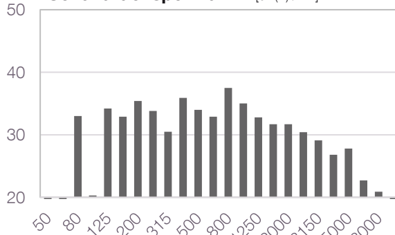
Schalldruckspektrum 6) [dB(A) / Hz]
