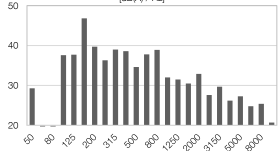
Spectre de pressions acoustiques 6) [dB(A) / Hz]
