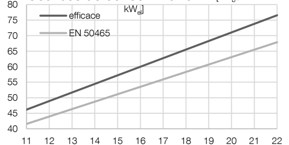
Courbes de consommation 3) [kW b / kW e ]
